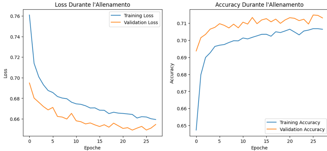
Figura III.3: Andamento della loss durante l'addestramento
