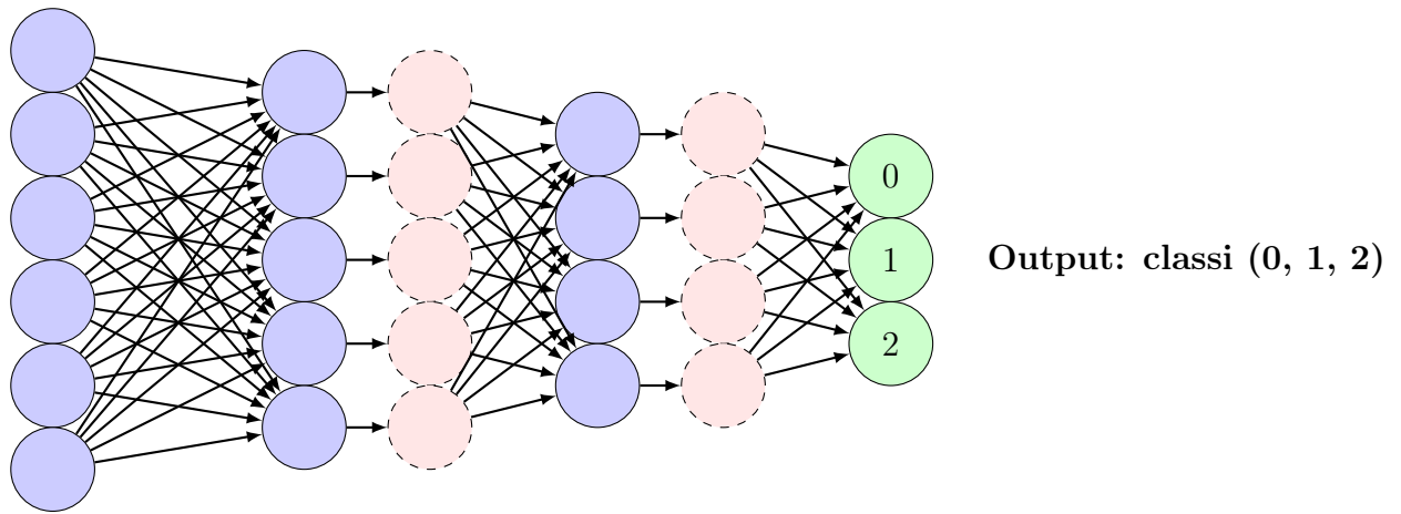
Figura III.2: Architettura della rete neurale con classi di output etichettate (0, 1, 2)
