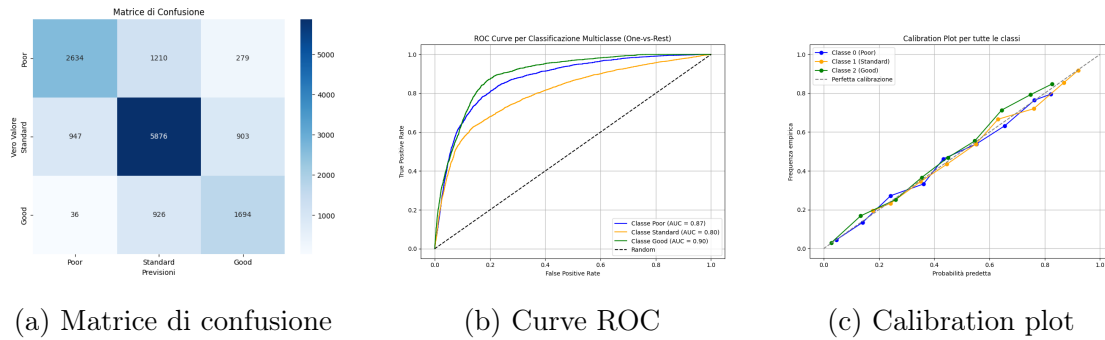
Figura III.4: Grafici di validazione dei risultati per la rete neurale
