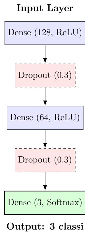
Figura III.1: Schema visivo dell'architettura della rete neurale
