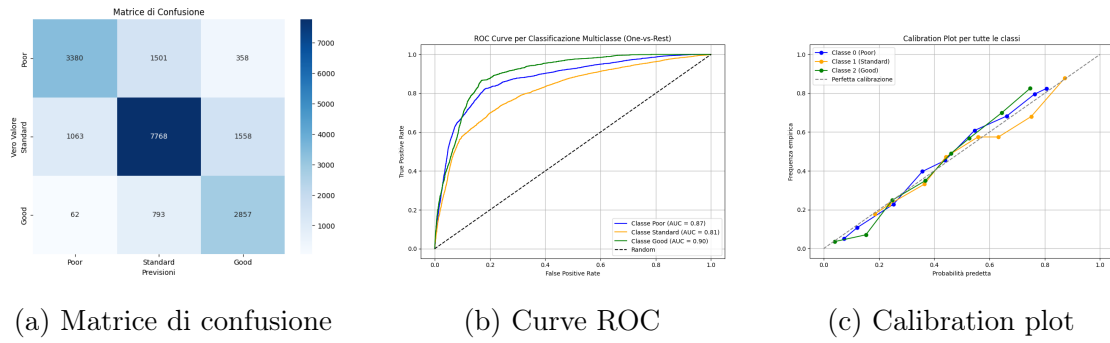
Figura III.5: Grafici di validazione dei risultati per la random forest
